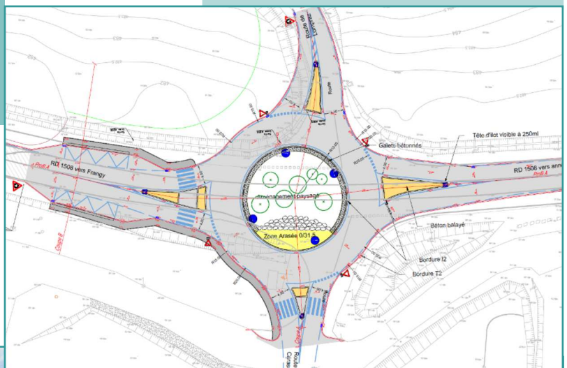
Plan Projet du Giratoire
